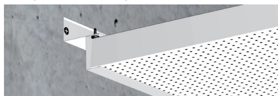
Rive joint creux réglable en deux éléments
