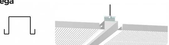
Porteur acier Omega
