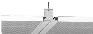
Porteur aluminium GAUGUIN 2 ou acier Rail C joint creux
